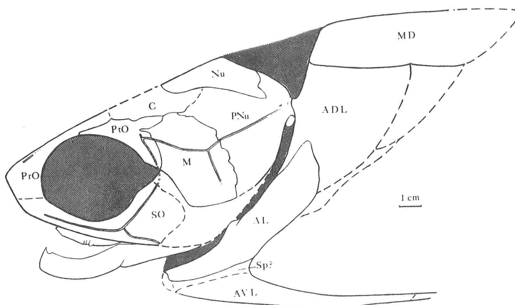
Fig. 5. - Reconstitution de l'ensemble des cuirasses dermiques de Melanosteus occitanus gen. et sp. nov., en vue latérale gauche.
