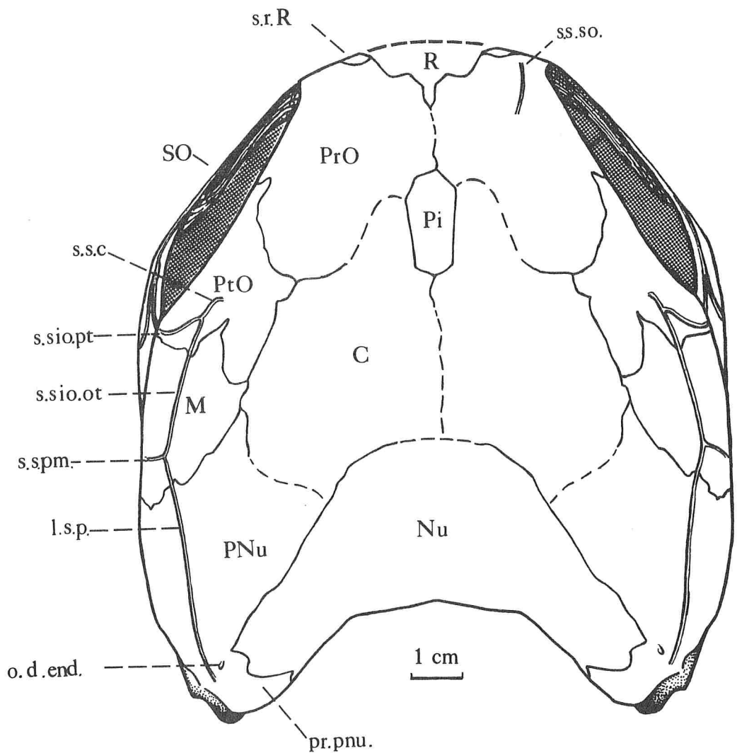
Fig. 2. - Reconstitution du toit crânien de Melanosteus occitanus gen. et sp. nov., en vue dorsale.
