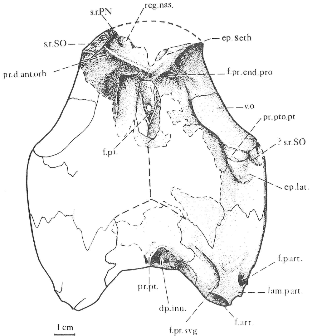
Fig. 3. - Interprétation de la face ventrale du toit crânien de Melanosteus occitanus gen. et sp. nov.
