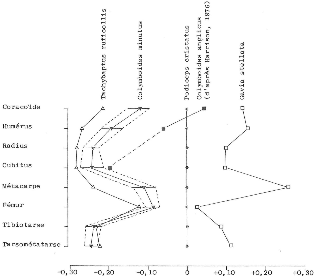
Fig. 2. — Diagramme de Simpson comparant la longueur totale des principaux segments osseux de Colymboides minutus , C. anglicus et des genres actuels Gavia (Gaviiformes) et Tachybaptus et Podiceps (Podicipediformes). (Pour C. minutus , le triangle représente la longueur moyenne et les traits de part et d'autre la variation extrême).
