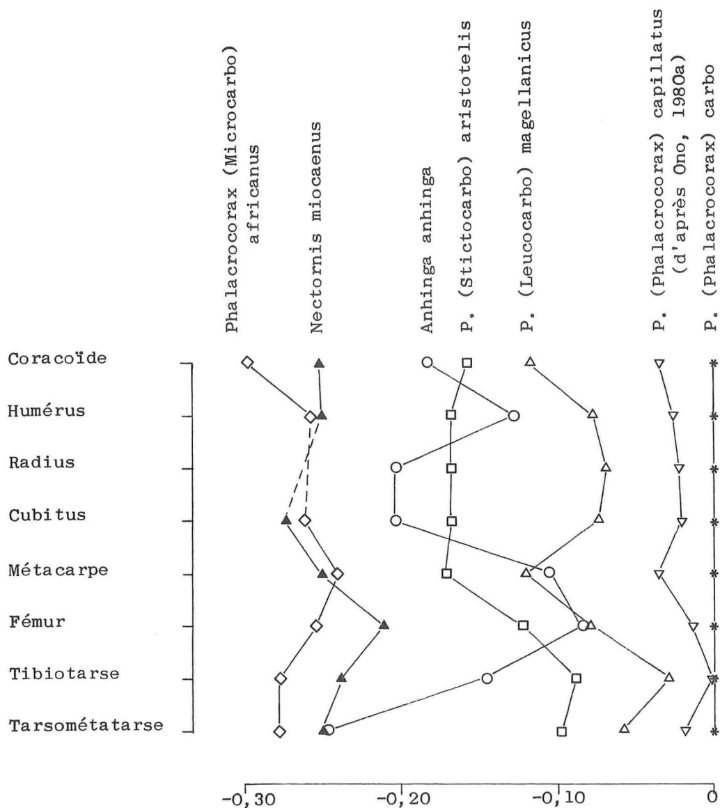
Fig. 3. — Diagramme de Simpson comparant la longueur totale des principaux segments osseux de Nectornis miocaenus et des genres actuels Phalacrocorax et Anhinga .
