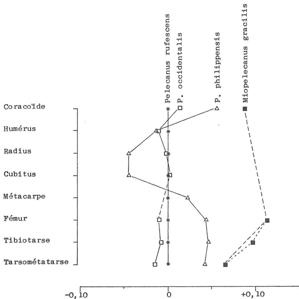
Fig. 4. — Diagramme de Simpson comparant la longueur totale des principaux segments osseux de Miopelecanus gracilis et du genre actuel Pelecanus . (La longueur du tibiotarse de M. gracilis est estimée).
