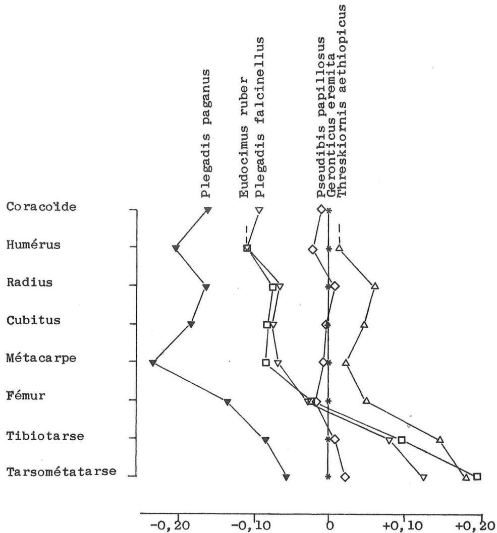
Fig. 5. — Diagramme de Simpson comparant la longueur totale des principaux segments osseux de Plegadis paganus et des genres actuels Plegadis , Eudocimus , Pseudibis , Geronticus et Threskiornis .
