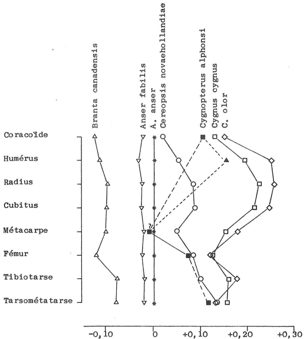
Fig. 6. — Diagramme de Simpson comparant la longueur totale des principaux segments osseux de Cygnopterus alphonsi et des genres actuels Branta , Anser , Cereopsis et Cygnus . (Le triangle noir représente l'humérus de Cygnopterus affinis ).
